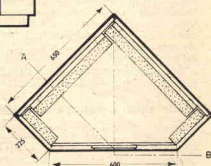
Fig. 2 - Mobile acustico pentagonale adatto a contenere due altoparlanti al alta fedeltà, del diametro di circa 220 mm. Ad esempio: PHILIPS HI-FI 9710 (campo di frequenza 40-10.000 HZ) PHILIPS BICONO n. 9710 M (campo di frequenza 40-20.000 Hz).
