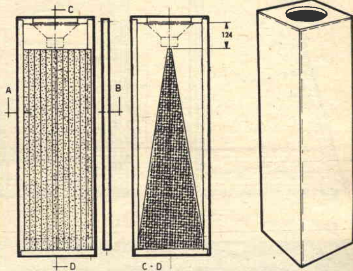
Fig. 7 - MOBILE ACUSTICO TIPO BASS-REFLEX particolarmente adatto per altoparlanti HI-FI normali o bifonici del diametro di 220/230 mm, ad esempio: PHILIPS HI-FI n. 9710 (campo di frequenza 40-10.000 Hz) PHILIPS BIFONICO n. 9710 M (campo di frequenza 40-20.000 Hz). N.B. Si tenga presente di tenere distanziati dalle pareti interne del mobile i pannelli assorbenti di circa 7-10 mm.
