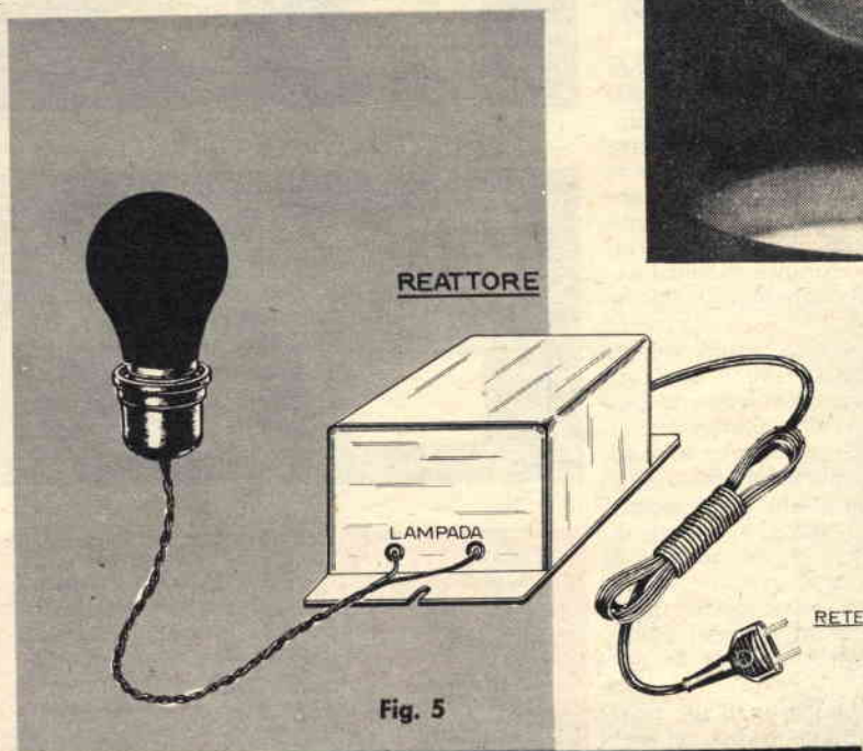
Fig. 5 - Installare una lampada di Wood è facilissimo; occorrono: un comune zoccolo portalampada, un reattore particolare, costruito appositamente per tale lampada, ed un cordone con spina. E' consigliabile, per evitare eventuali irritazioni agli occhi, completare l'installazione con un riflettore in metallo o cartone, in modo da dirigere la «luce» solo sugli oggetti o sostanze da controllare.
