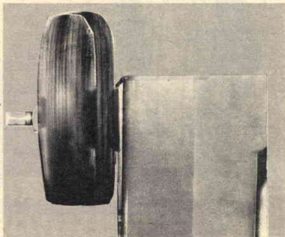
Fig. 7 - Quando la ruota è squilibrata, anche a medie velocità tende ad oscillare lateralmente. Nella foto la fotografia effettuata con uno stroscopio durante la fase oscillante.
