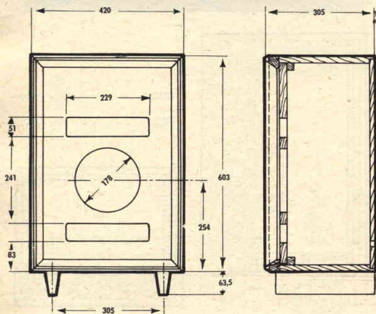
Fig. 10 - Mobile acustico BASS-REFLEX adatto a ricevere altoparlanti HI-FI o bifonici con diametro compreso tra i 200 e i 220 mm. Tale mobile di forma parallelepipedica, dispone sul pannello frontale di due aperture appositamente calcolate della lunghezza di 51 mm e della lunghezza di 229 mm. Tale mobile non richiede pannelli interni assorbenti.
