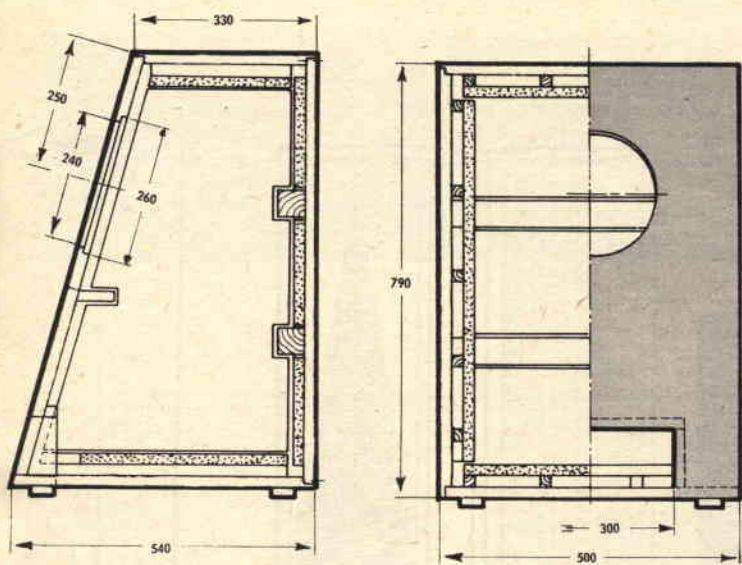
Fig. 8 - Dettagli costruttivi del mobile acustico BASS-REFLEX presentato a fig. 7 ed a fig. 9.
