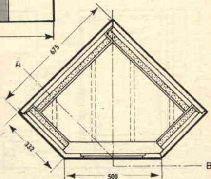
Fig. 3 - Mobile acustico pentagonale adatto per un altoparlante di 330 mm di diametro, ad esempio: PHILIPS HI-FI n. 9760 (campo di frequenza 50-10.000 Hz) PHILIPS BICONO n. 9760 M (campo di frequenza 35-10.000 Hz) PHILIPS HI-FI n. 9762 (campo di frequenza 60-8.000 Hz) PHILIPS BICONO n. 9762 M (campo di frequenza 40-19.000 Hz).
