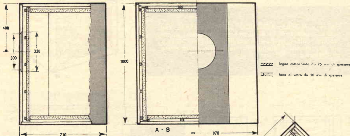
Fig. 3 - Mobile acustico pentagonale adatto per un altoparlante di 330 mm di diametro, ad esempio: PHILIPS HI-FI n. 9760 (campo di frequenza 50-10.000 Hz) PHILIPS BICONO n. 9760 M (campo di frequenza 35-10.000 Hz) PHILIPS HI-FI n. 9762 (campo di frequenza 60-8.000 Hz) PHILIPS BICONO n. 9762 M (campo di frequenza 40-19.000 Hz).
