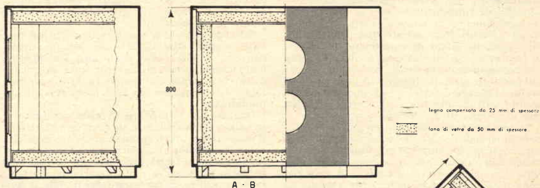
Fig. 2 - Mobile acustico pentagonale adatto a contenere due altoparlanti al alta fedeltà, del diametro di circa 220 mm. Ad esempio: PHILIPS HI-FI 9710 (campo di frequenza 40-10.000 HZ) PHILIPS BICONO n. 9710 M (campo di frequenza 40-20.000 Hz).
