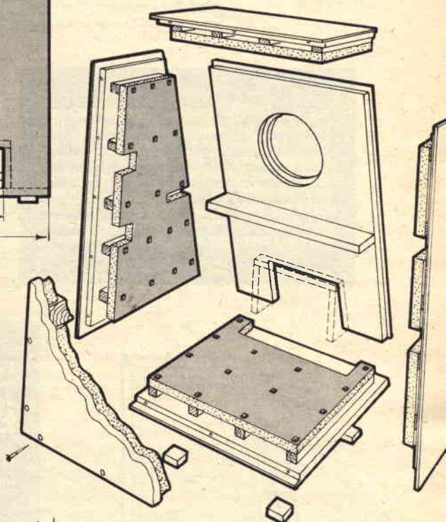
Fig. 8 - Dettagli costruttivi del mobile acustico BASS-REFLEX presentato a fig. 7 ed a fig. 9.
